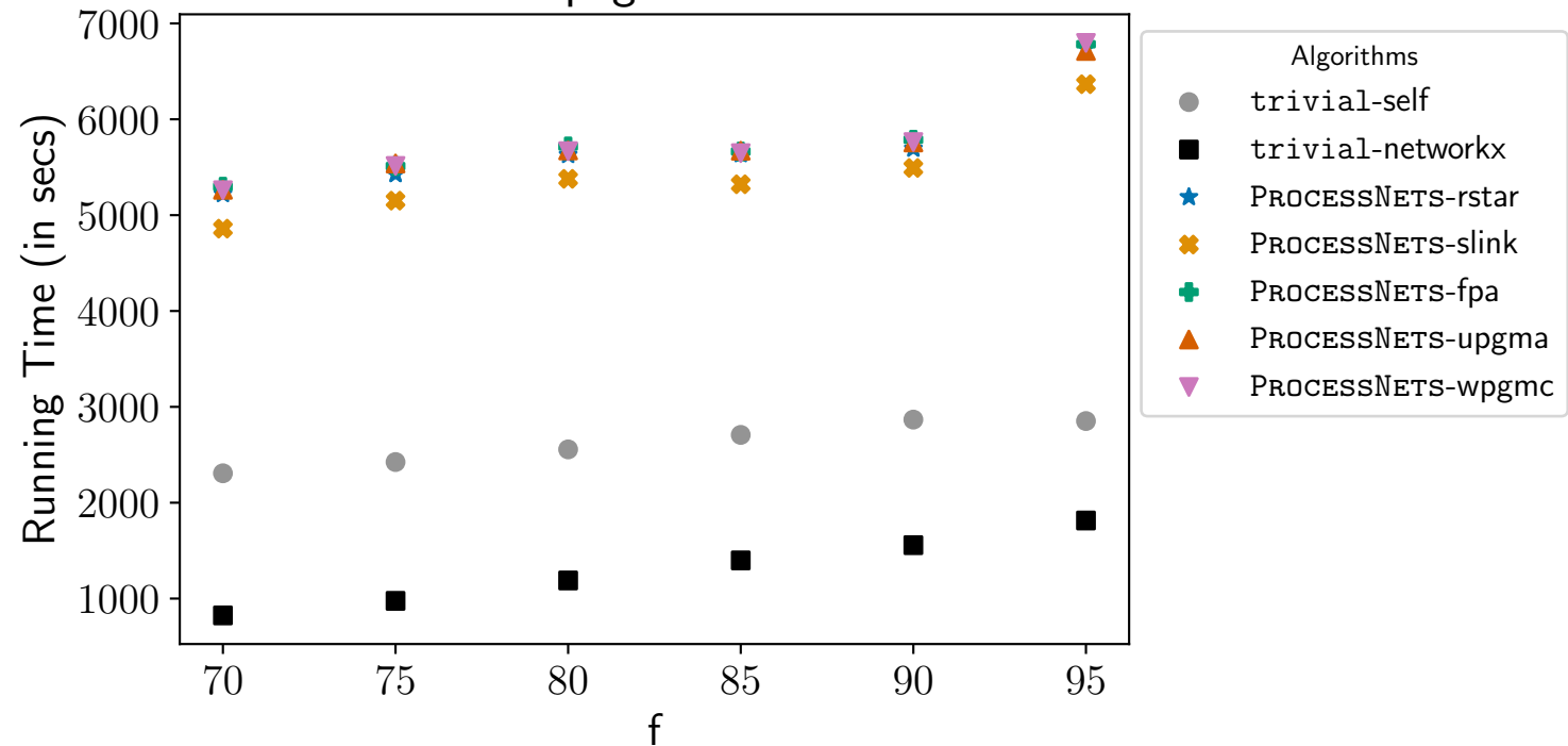
pagerank
